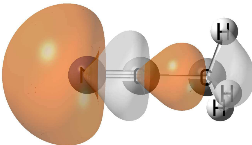
HOMO-1
